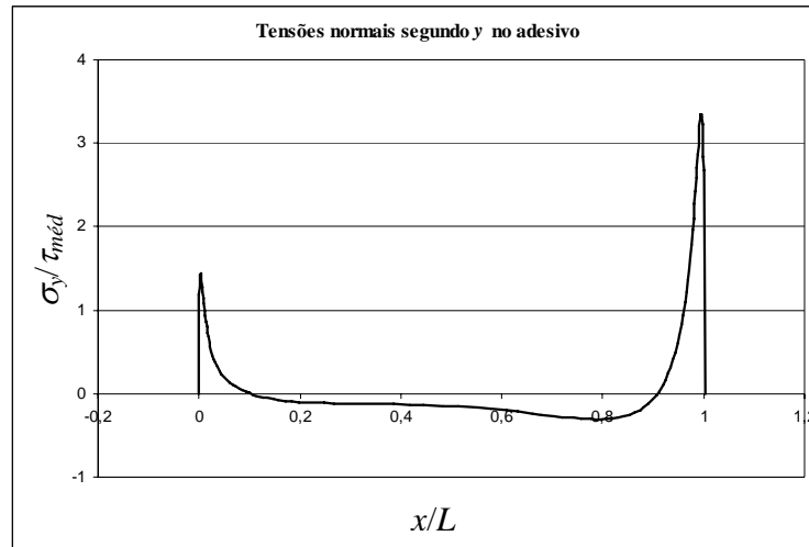
Fig. 3. Tensões normais segundo y no adesivo.
