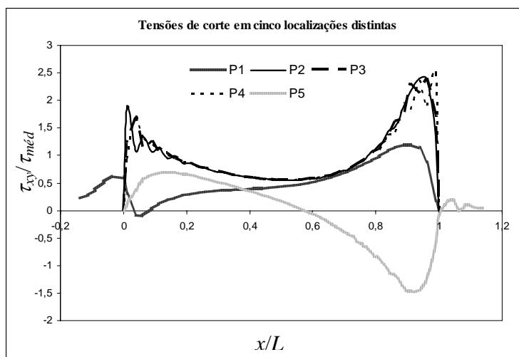
Fig. 7. Comparação das tensões de corte em cinco localizações distintas.
