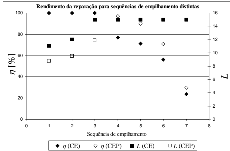
Fig. 23. Rendimento da junta colada em sobreposição dupla.
