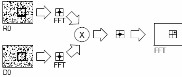
Fig. 4. Organograma do processamento efectuado na correlação digital de imagem.
