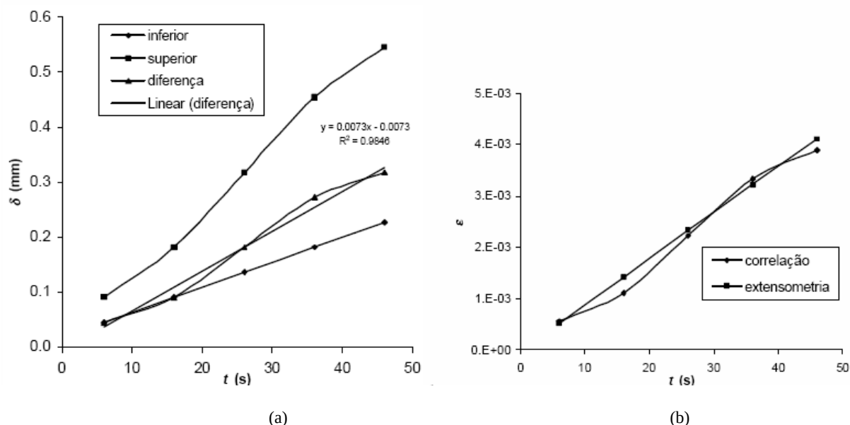
Fig. 10. (a) Deslocamentos obtidos em dois pontos nas extremidades visíveis do provete (90^\circ)_8 e respectiva diferença. (b) Comparação da deformação obtida pelos dois métodos utilizados.
