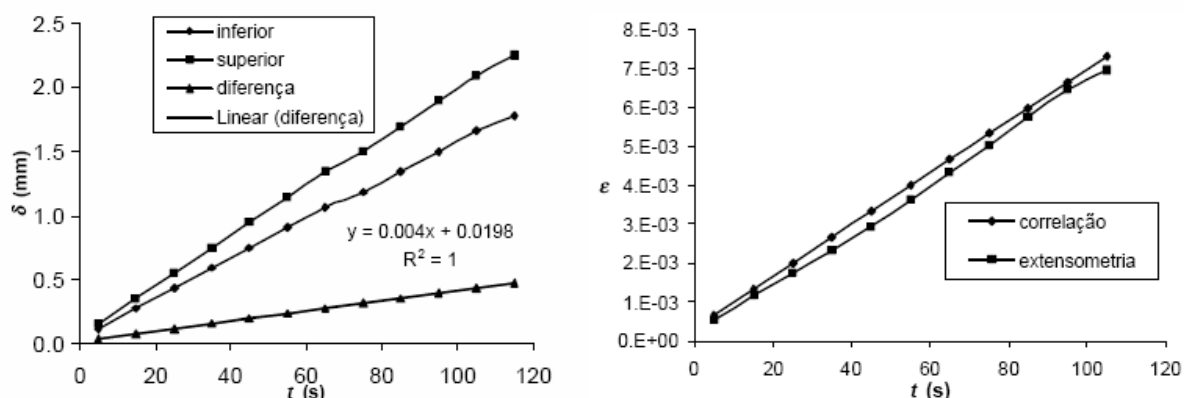
Fig. 9. (a) Deslocamentos obtidos em dois pontos nas extremidades visíveis do provete (0°) 8 e respectiva diferença. (b) Comparação da deformação obtida pelos dois métodos utilizados.
