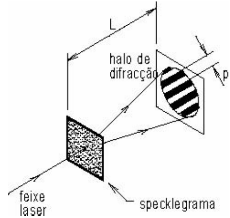
Fig. 2. Formação das franjas de Young na fotografia speckle .
