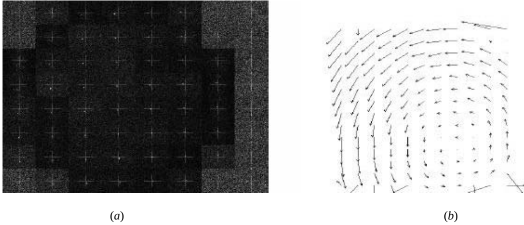
Fig. 6. Processamento da área completa da imagem de um objecto submetido a uma rotação. (a) Amostragem das correlações obtidas e (b) respectivo campo de deslocamentos no plano.
