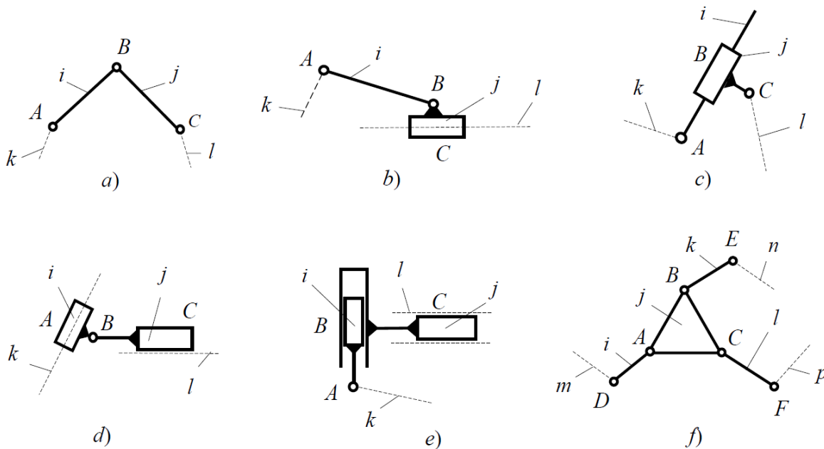
Fig. 2. Grupos estructurales de Assur de a) a e) son de segunda clase y f) es de tercera clase. Además, los de segunda clase se dividen en variedades. Estas son: a) de primera variedad; b) de segunda variedad; c) de tercera variedad; d) de cuarta variedad y e) de quinta variedad.
