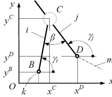
Fig. 5. Esquema de un grupo estructural convencional.
