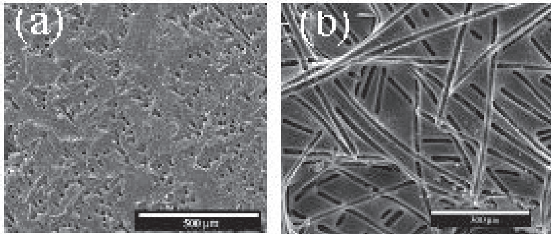
Fig. 2. Microscopia de barrido: (a) vista superior. (b) vista lateral de muestras con conductos capilares obtenidos despues de la carbonización de las fibras.
