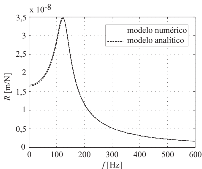
Fig. 9. Comparación de la receptancia vertical de la vía DFF determinada con los modelos numérico y analítico.
