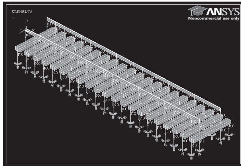
Fig. 6. Modelo numérico de vía convencional completa sobre balasto.
