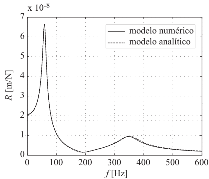
Fig. 10. Comparación de la receptancia vertical de la vía bloqueada con los modelos numérico y analítico.
