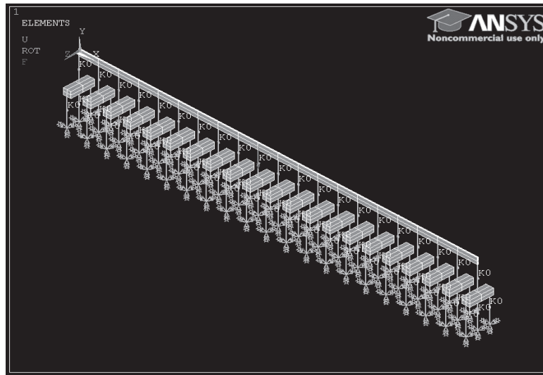
Fig. 5. Modelo numérico de media vía bibloque.
