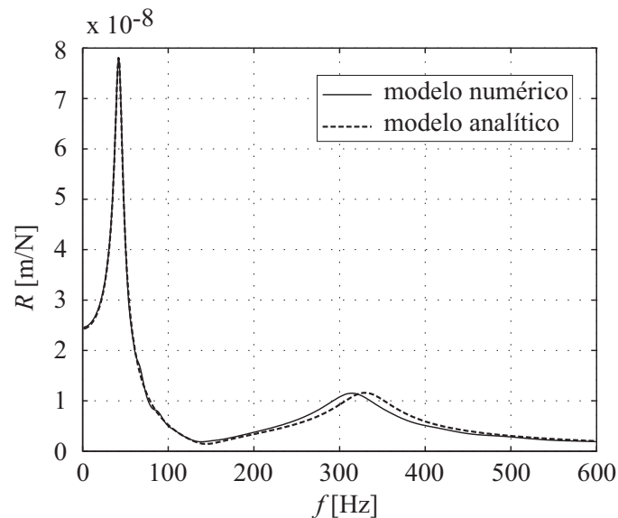
Fig. 11. Comparación de la receptancia vertical de la vía convencional con el modelo numérico completo y el modelo analítico de media vía.
