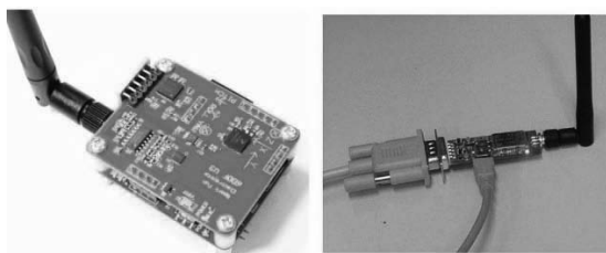
Fig. 2. Plataforma inercial Sparkfun constituída de circuito transmissor com sensores (esquerda) e circuito receptor (direita).
