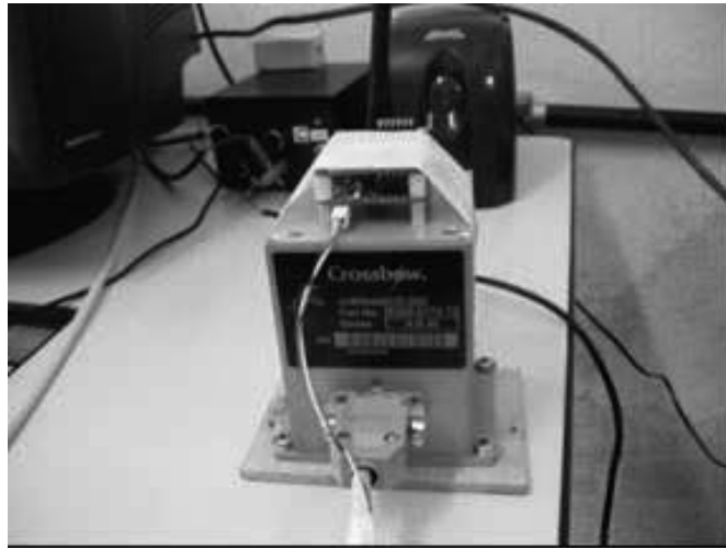
Fig. 5. Plataformas Crossbow e Sparkfun fixadas para calibração.
