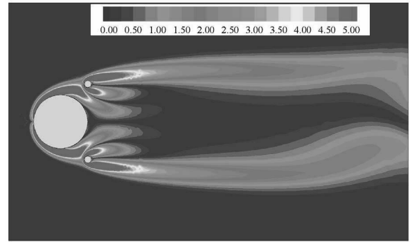
Fig. 8. Topologia do escoamento e vorticidade para (Xc/D=0.5, Yc/D=0.5) .
