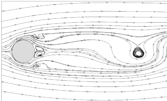
Fig. 8. Topologia do escoamento e vorticidade para (Xc/D=0.5, Yc/D=0.5) .
