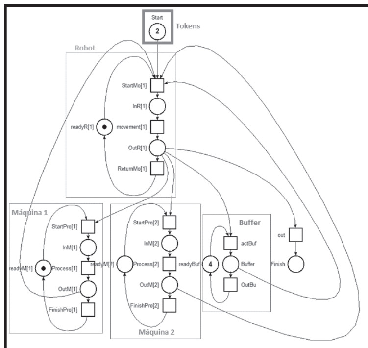
Fig. 2. Redes de Petri para Simulador Gráfico.
