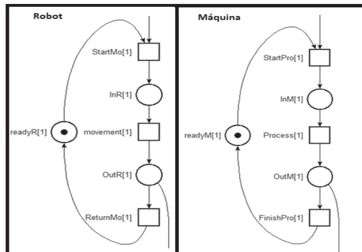
Fig. 1. Redes de Petri para Máquina y Robot.
