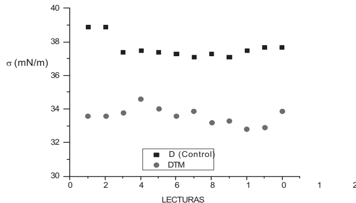
Fig. 5. Tensión superficial de las muestras de diésel antes (D) y después del tratamiento magnético (DTM).
