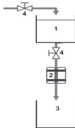
Fig. 2. Esquema del tratamiento magnético del combustible. (1-Recipiente con diésel, 2-Acondicionador magnético, 3-Vaso de precipitado, 4-Válvulas).
