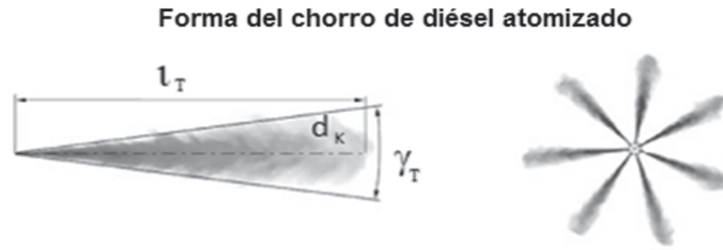
Fig. 6. Parámetros del chorro de combustible atomizado ( l_T – profundidad de penetración del chorro, d_K – diámetro medio de las gotas en el chorro, \gamma_T – ángulo de apertura del chorro).
