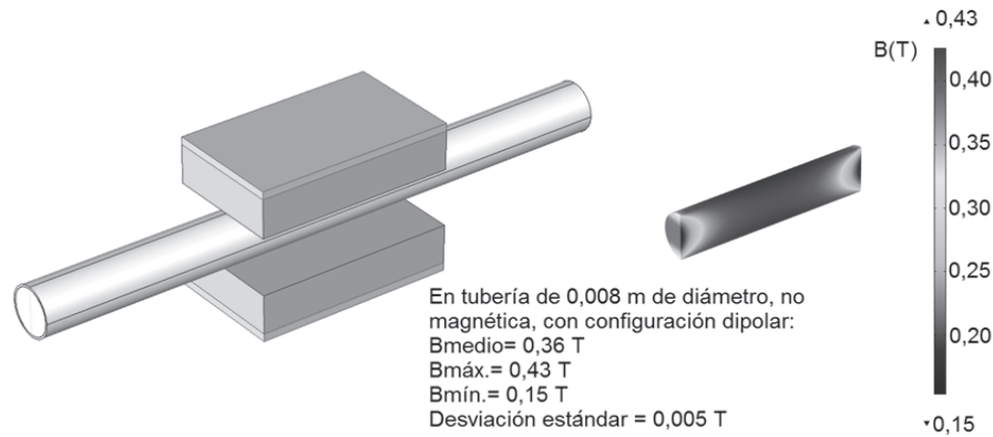
Fig. 1. Patrón de distribución de campo magnético en una tubería diamagnética (B-inducción magnética, B_{\text{máx.}} - inducción máxima, B_{\text{mín.}} - inducción mínima).
