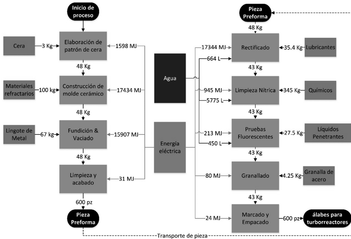
Fig. 3. Diagrama cuantitativo del proceso de fabricación.
