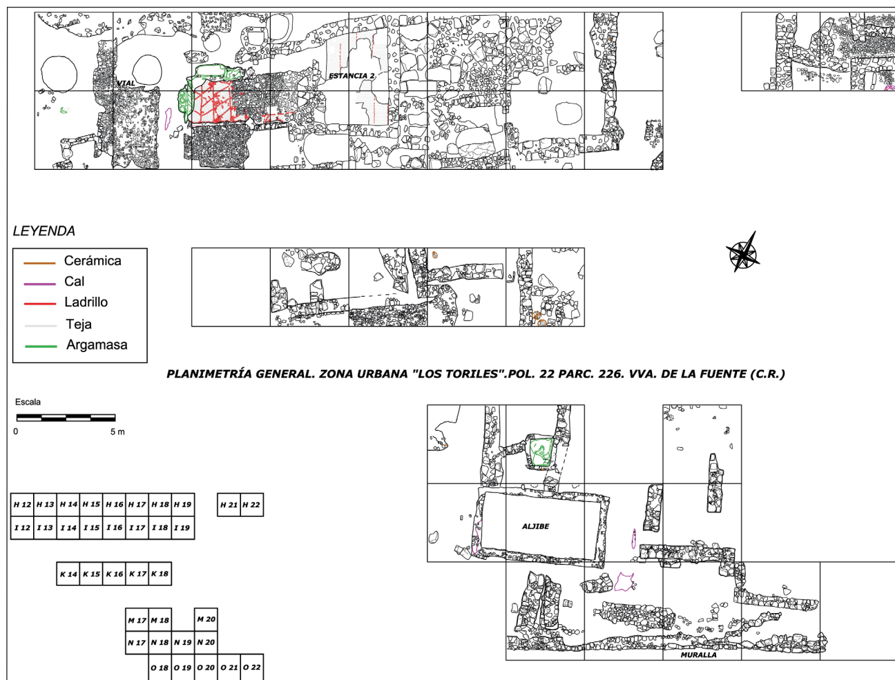
▲ FIGURA 3. Planta general del área urbana de Mentesa Oretana estudiada en "Los Toriles".
